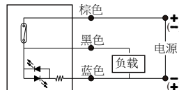
磁簧管3线
