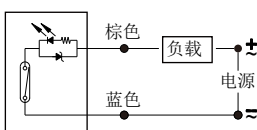
磁簧管2线
