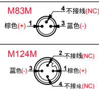
接头2线
