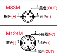
接头3线
