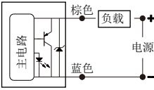
电子式2线
