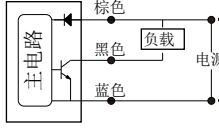
NPN型
