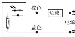
磁簧管2线
