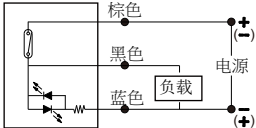
磁簧管3线
